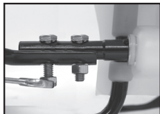
Figure 4 Serrez les écrous aux boulons
